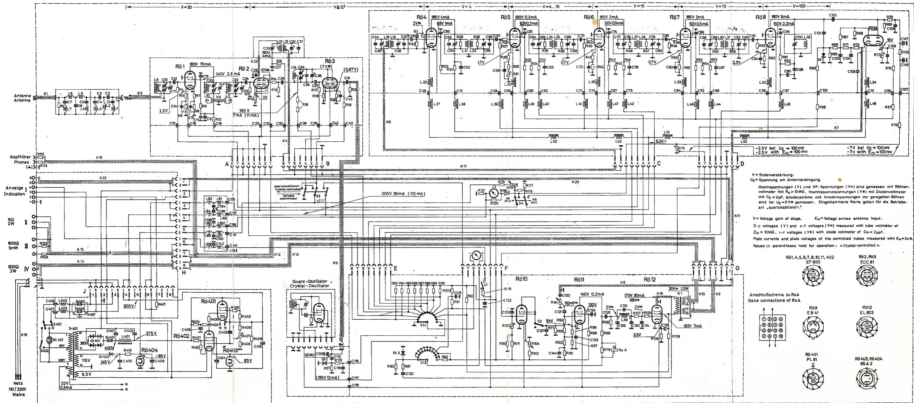
Bild 2. Stromlauf zum Flugsicherungsempfänger Type NE 1
